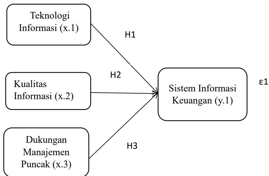
Gambar 1: Rerangka Konseptual
